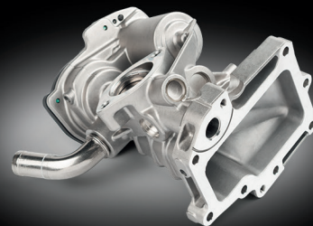
Клапан EGR Евро 5
